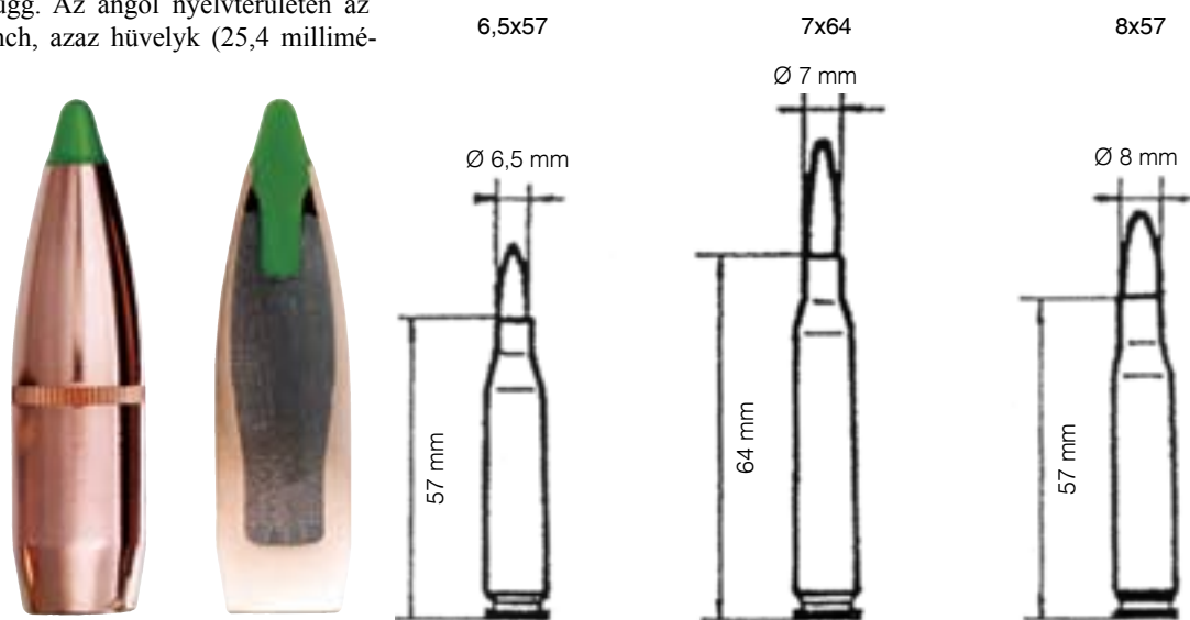
Golyós lőszer jellemző méretei
